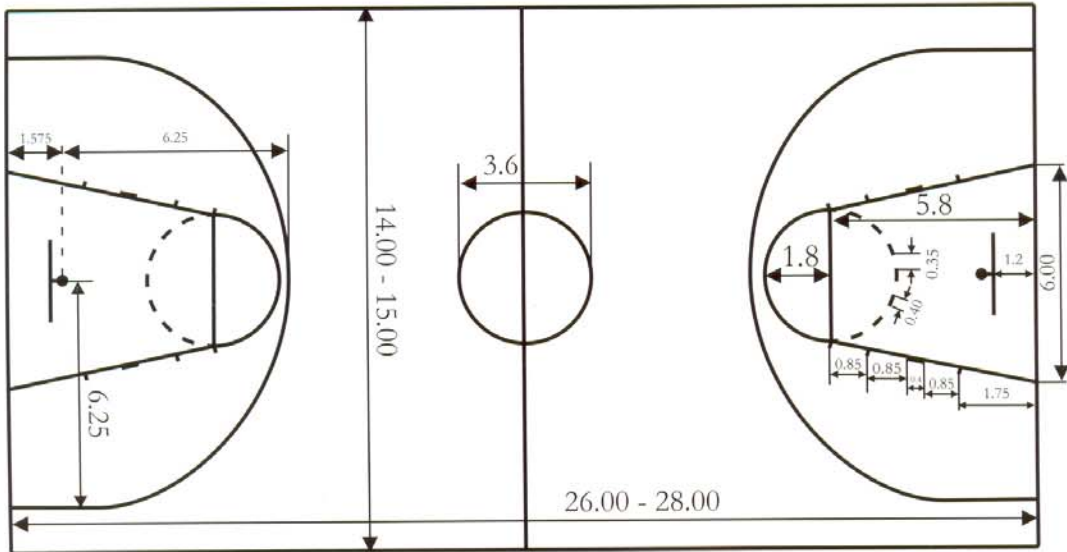
Разметка баскетбольной площадки.
