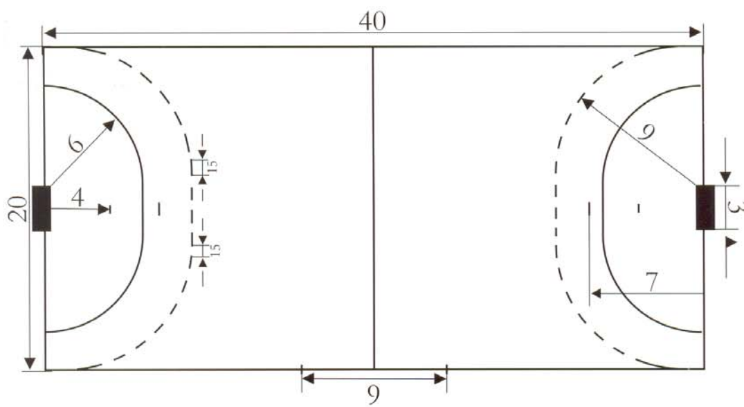
Разметка гандбольной площадки.
